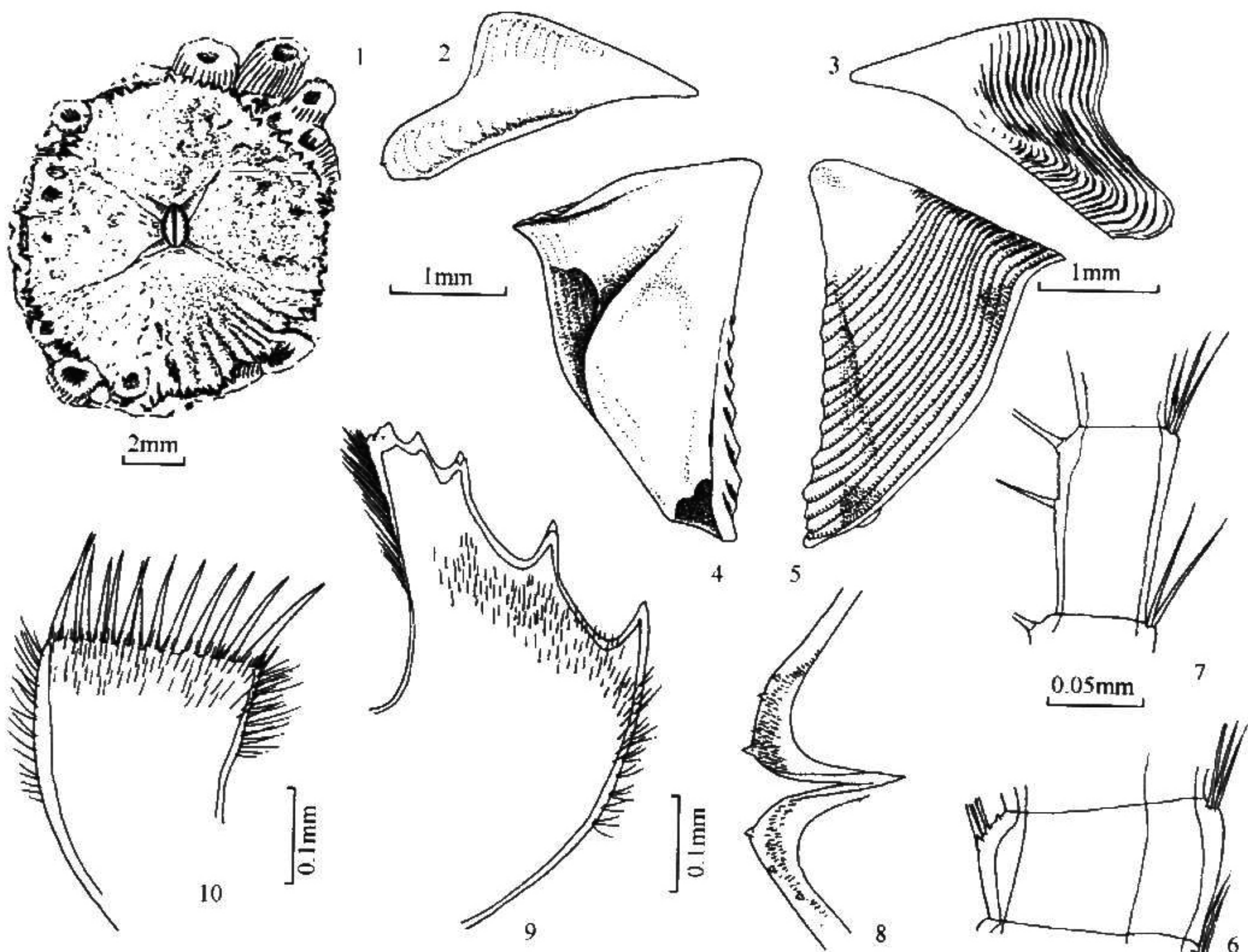
图 202 华离板藤壶 Cantellius sinensis Ren
